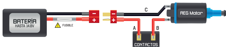
FIG 1. INSTALACIÓN AEG ESTÁNDAR
