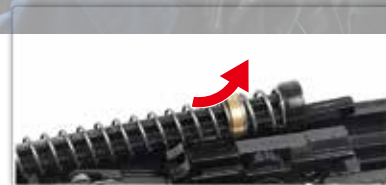
Avec précaution faites pivoter le guide de ressort et retirez-le lentement.
