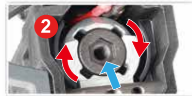
2.使用内六角(6mm)内壓尾頂桿之後轉動至開口處。
