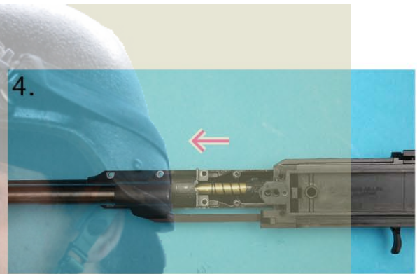
4) 分開前部 Detach the front assembly
