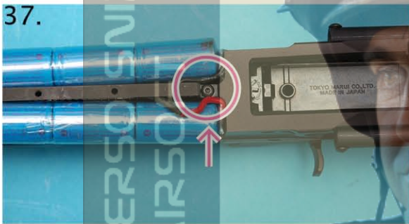
37) 電線在下方 Battery cords face downward
