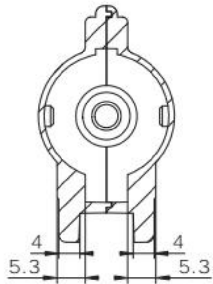
G2 GEARBOX
