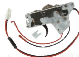
APE Lower Gearbox APE 下齒輪箱 MA-289
