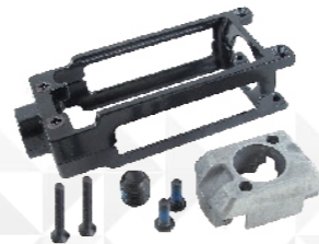
CES-P Motor Shell CES-P 馬達座組
